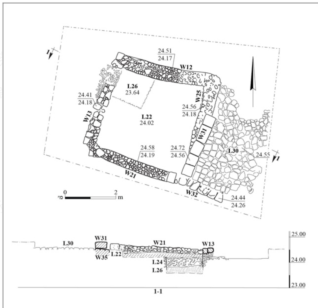
圖 4：B 區平面圖
