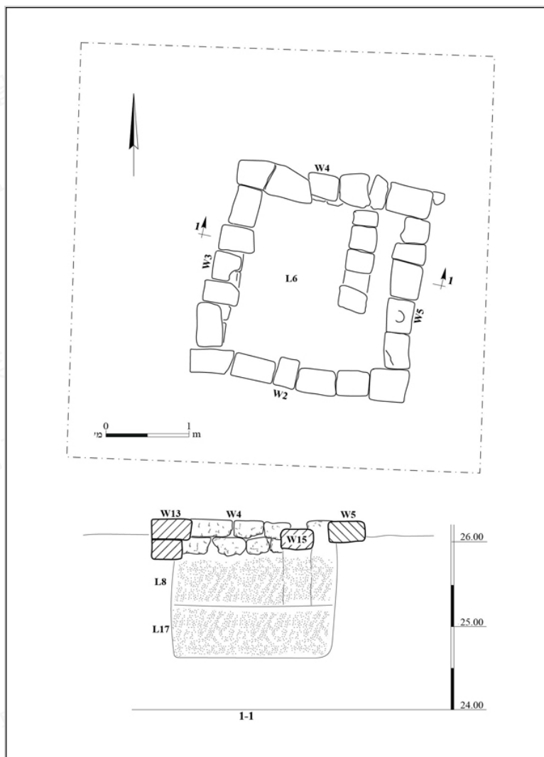
圖 7：D 區建築平面圖
