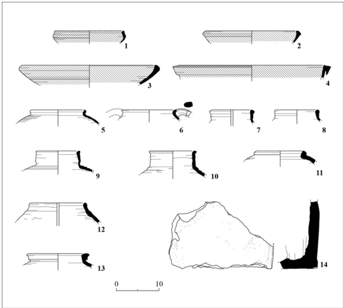
圖 6：B 區出土陶器與空心磚繪圖
