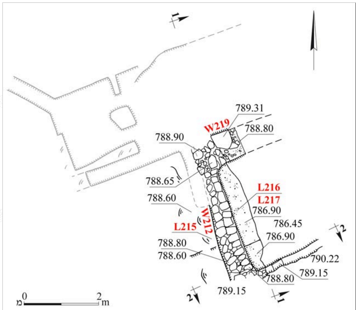
圖 13 : Pool (Stratum 2), plan.
