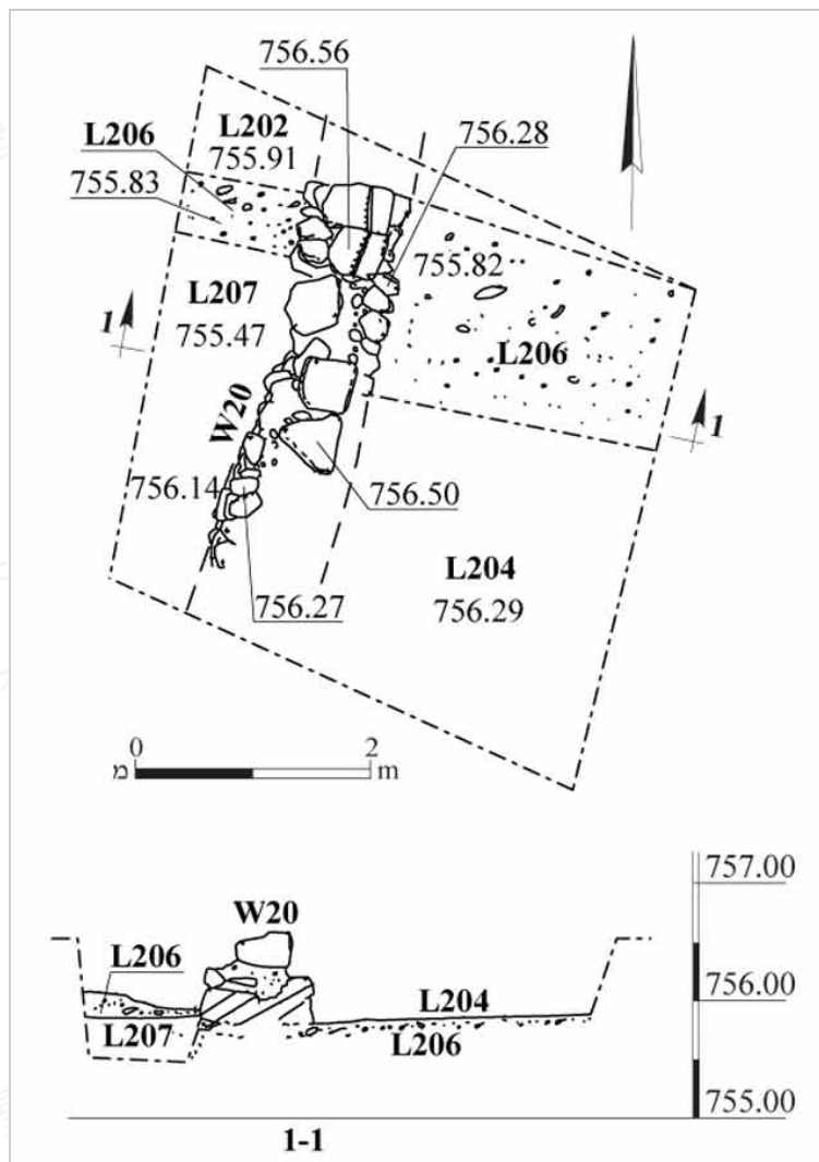
圖 3 : Area B, plan and section.
