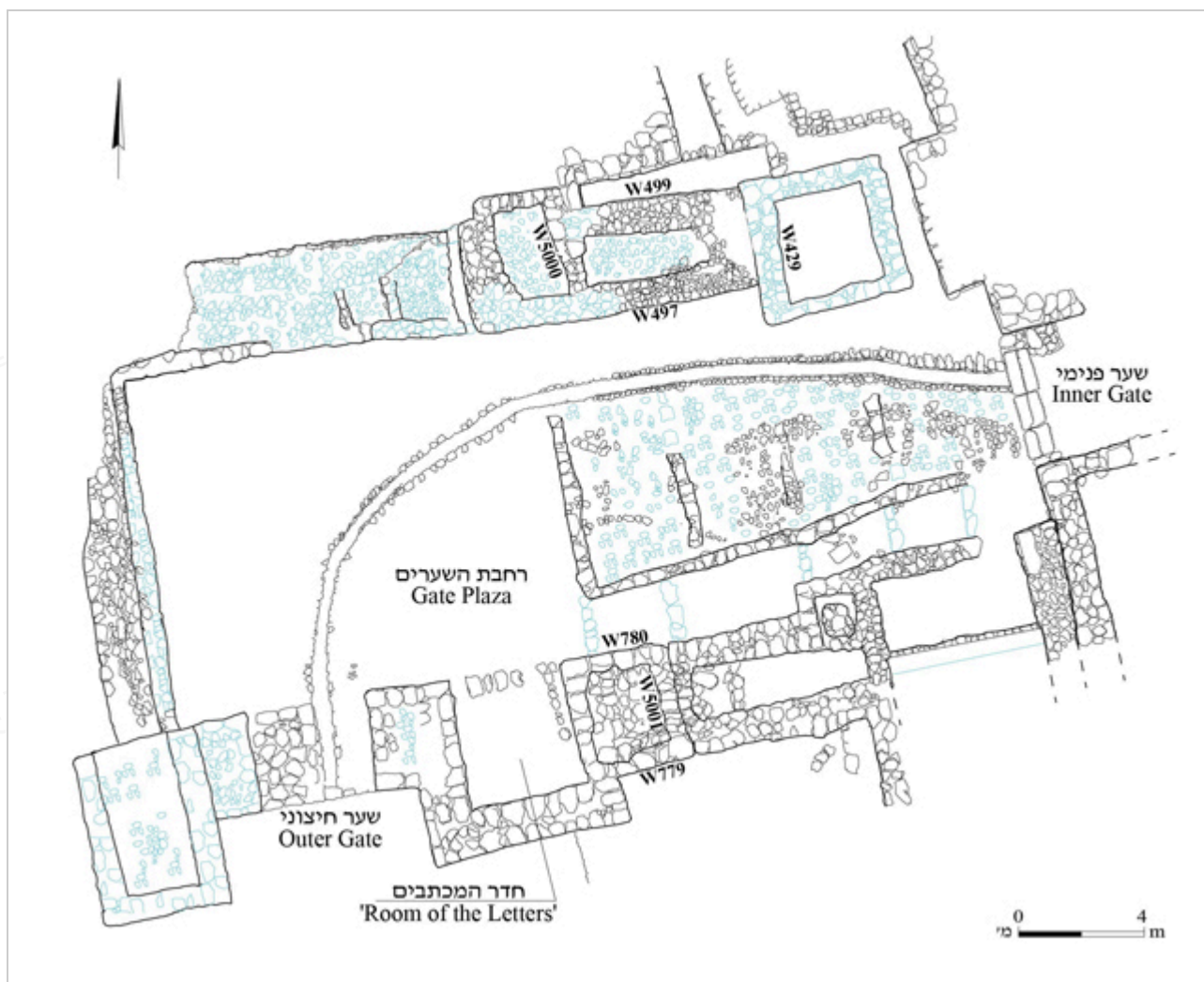
圖 3：平面圖
