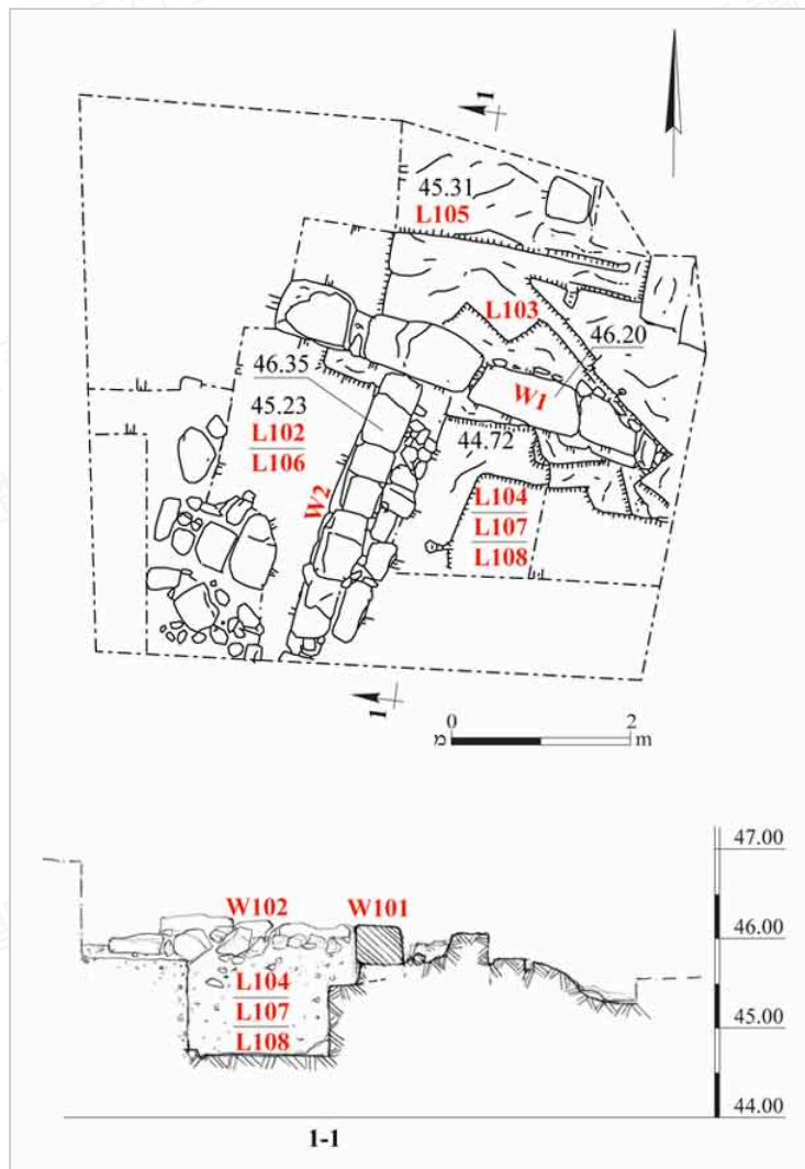
圖 1：平面圖與剖面圖
