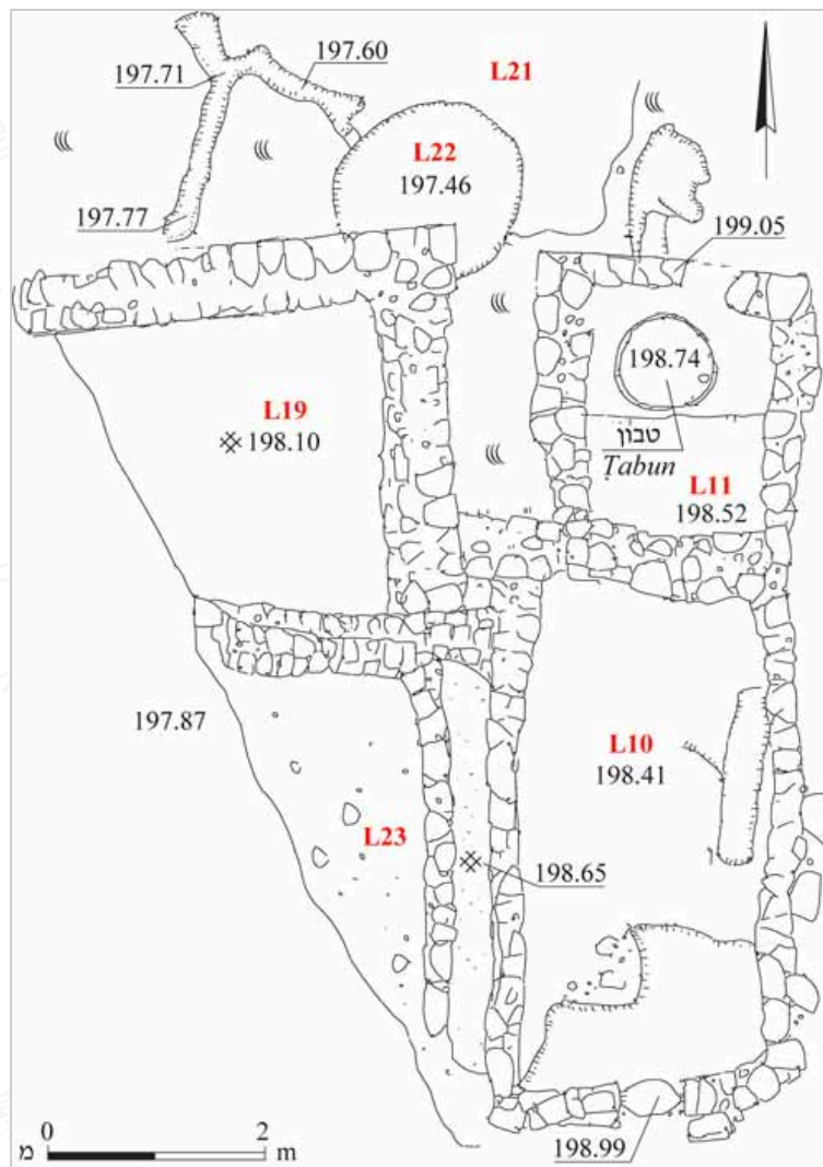
圖 8：第 54 號遺址，建築平面圖
