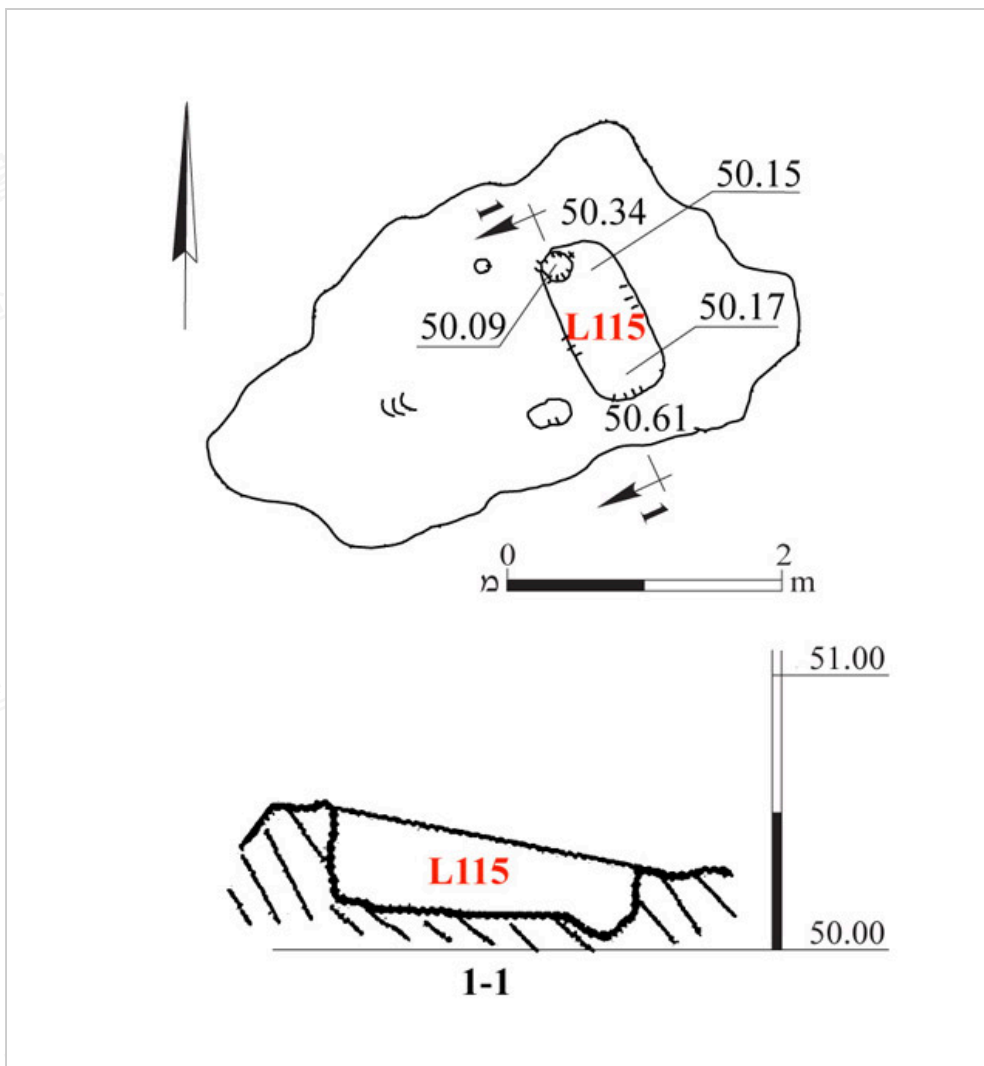
圖 14：榨酒池 7，平面圖與剖面圖
