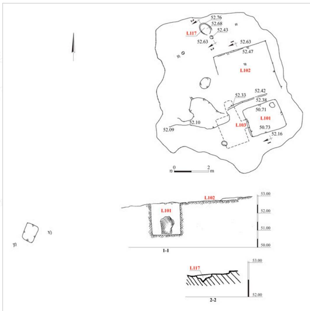
圖 3：榨酒池 1 與 5，平面圖與剖面圖
