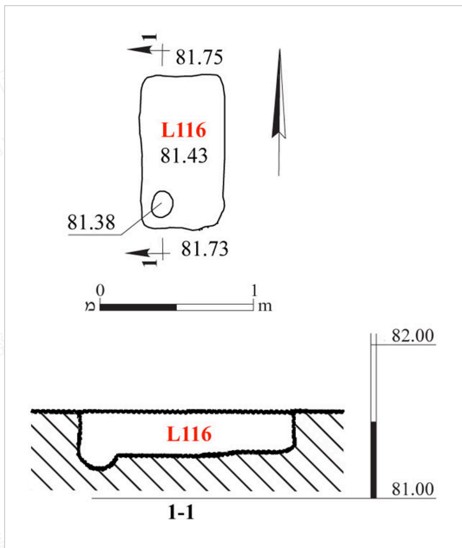
圖 16：榨酒池 8，平面圖與剖面圖
