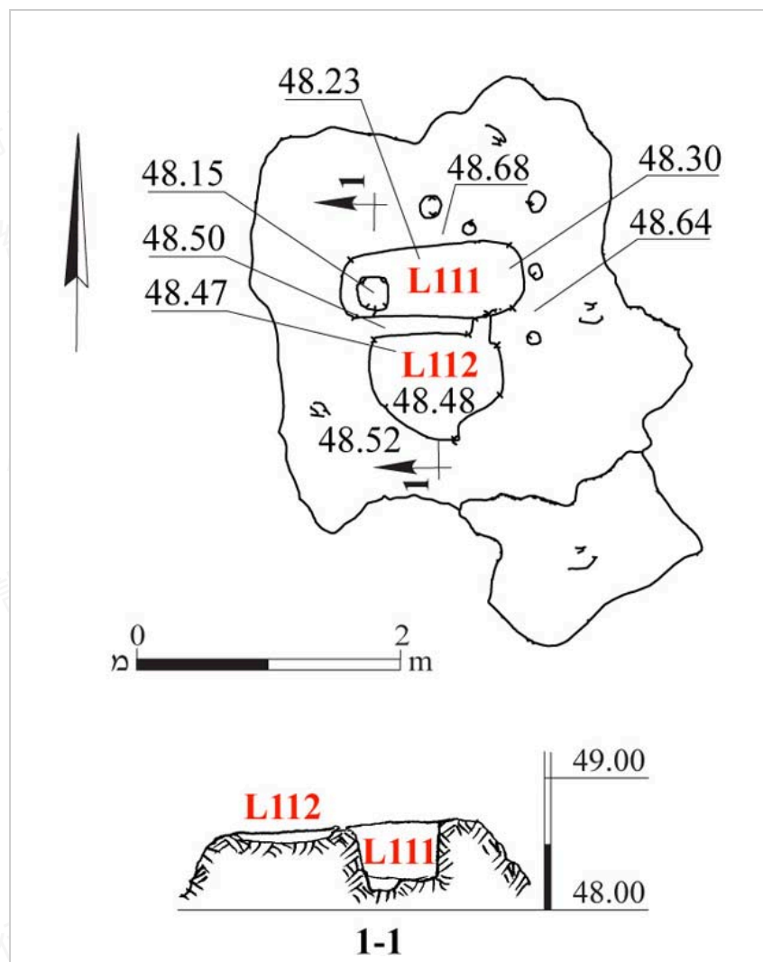
圖 10：榨酒池 4，平面圖與剖面圖
