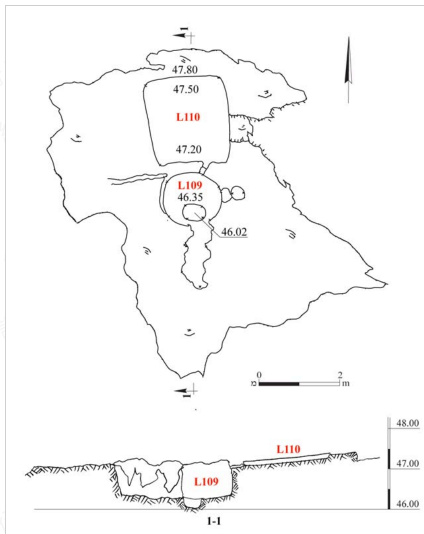
圖 8：榨酒池 3，平面圖與剖面圖
