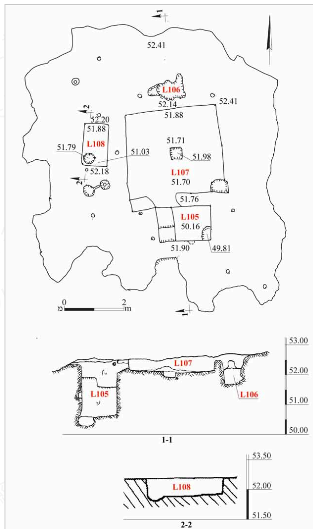
圖 6：榨酒池 2 與 6，平面圖與剖面圖
