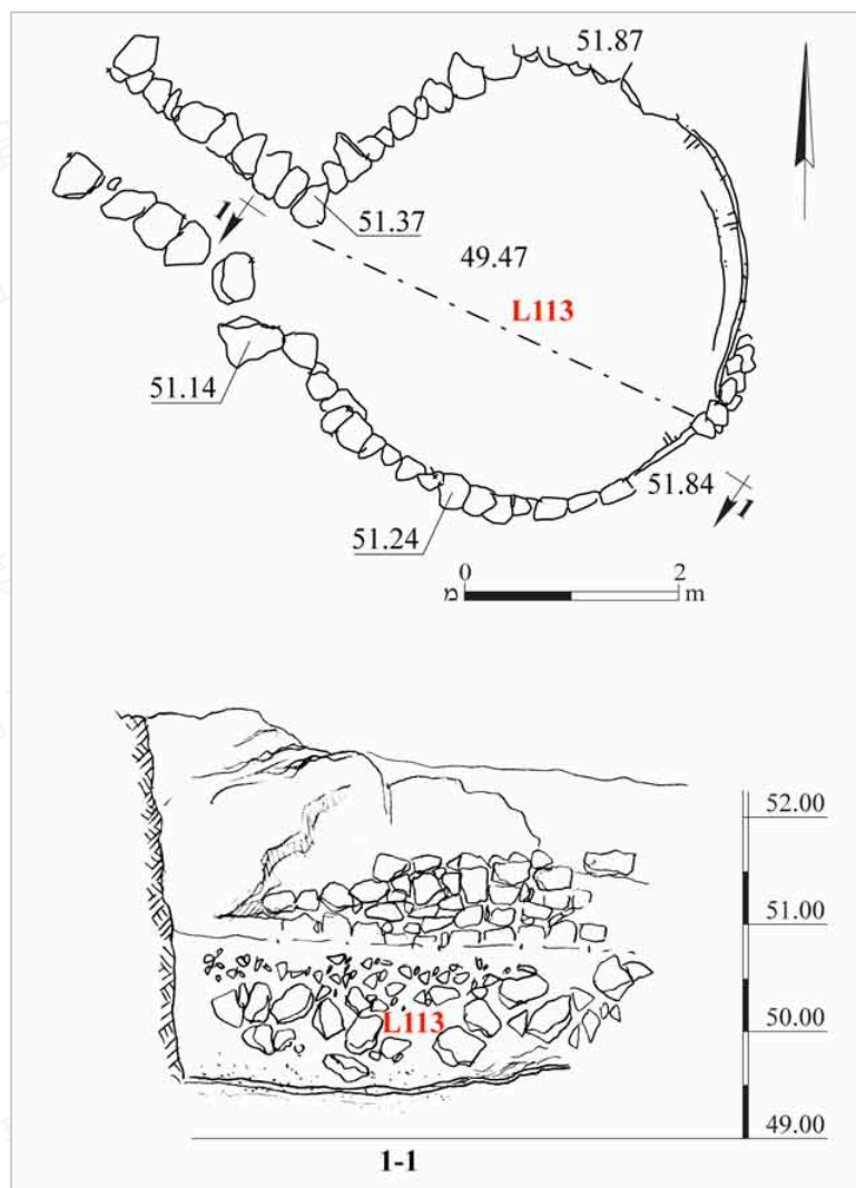
圖 18：石灰窯，平面圖與剖面圖
