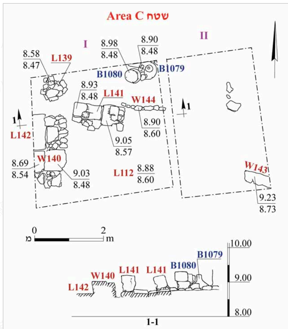
圖 3：C 區平面圖與剖面圖。
