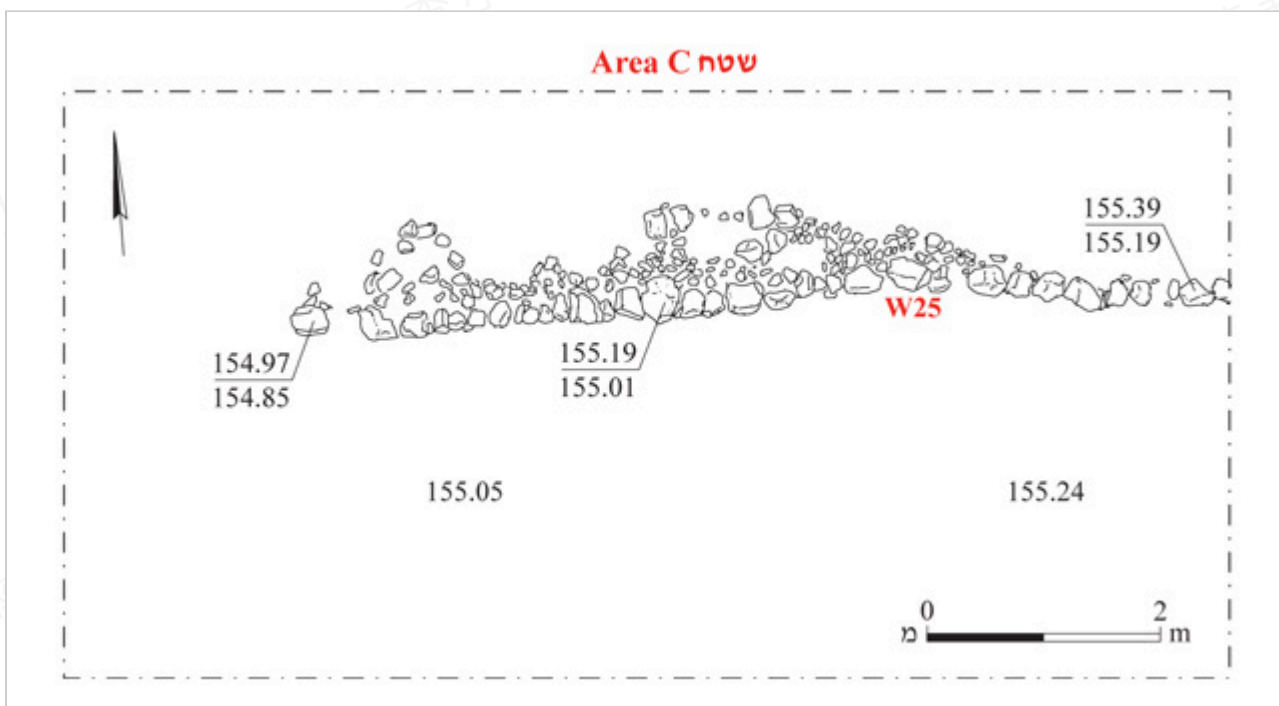
圖 8：C 區平面圖
