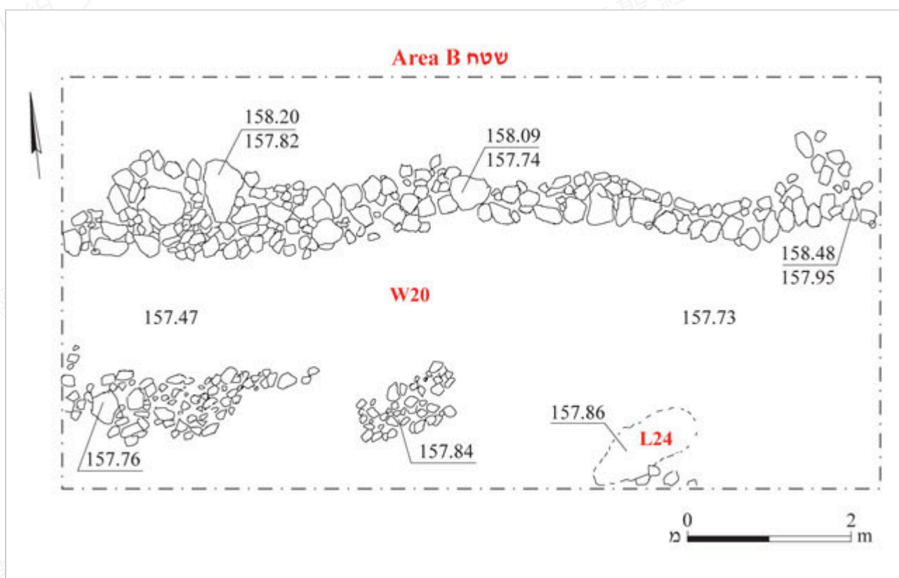
圖 6：B 區平面圖
