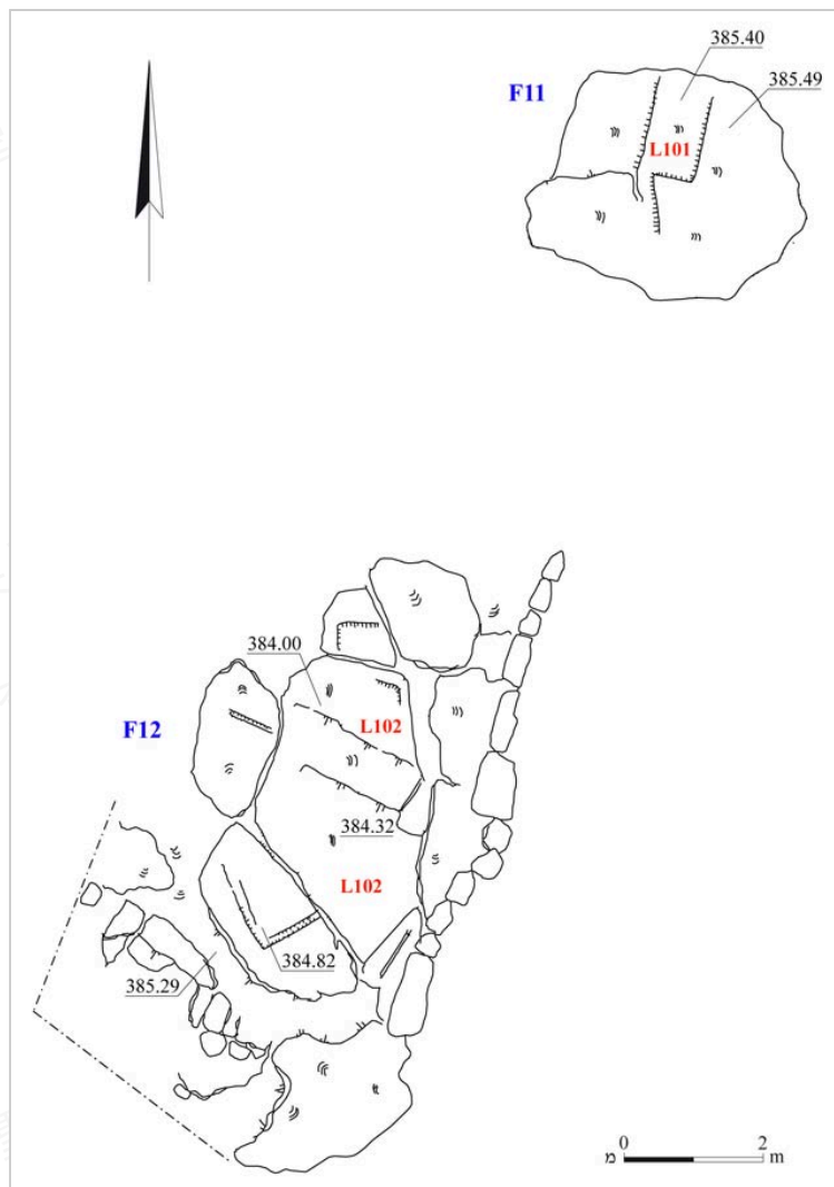
圖 12：F11 及 F12 採石場，平面圖
