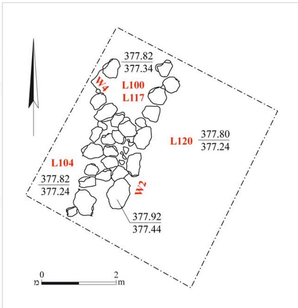
圖 6：F6 農耕圍籬 2 平面圖
