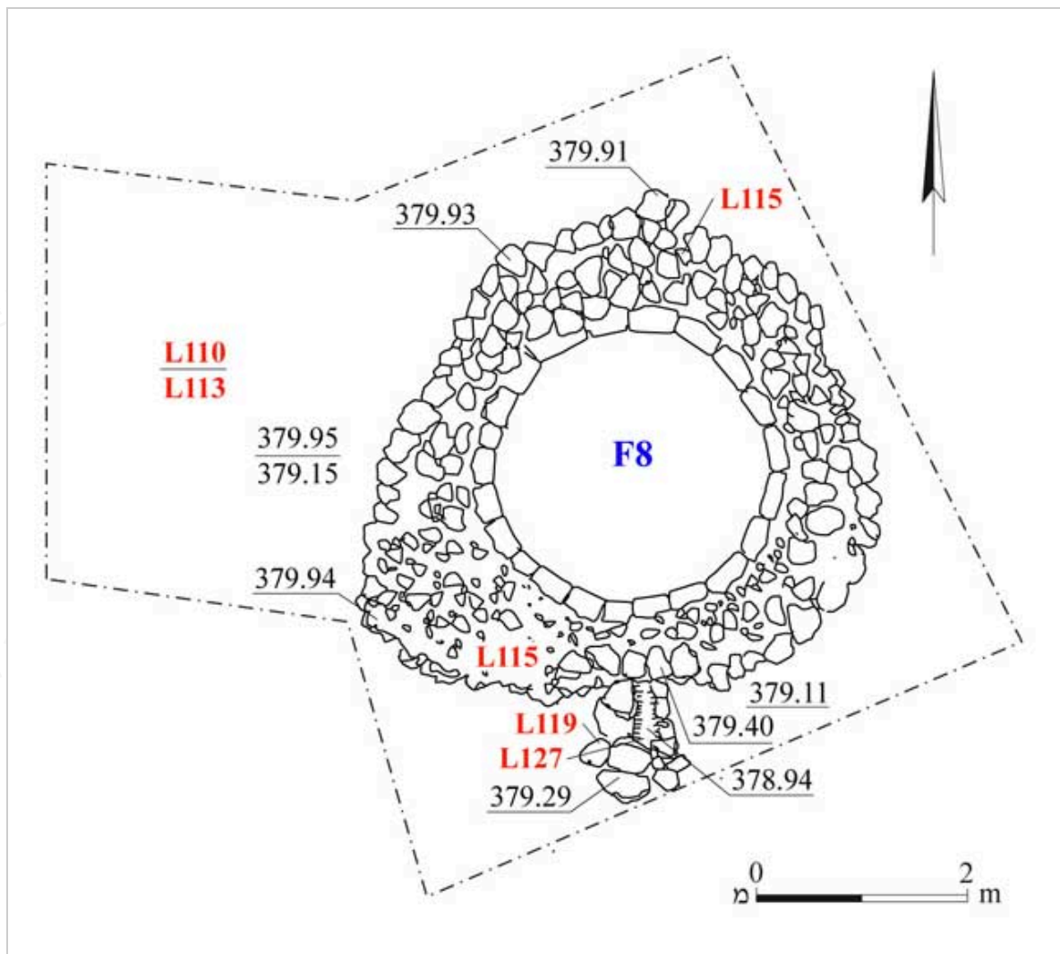
圖 10：F8 水井及石板覆蓋的水渠，平面圖
