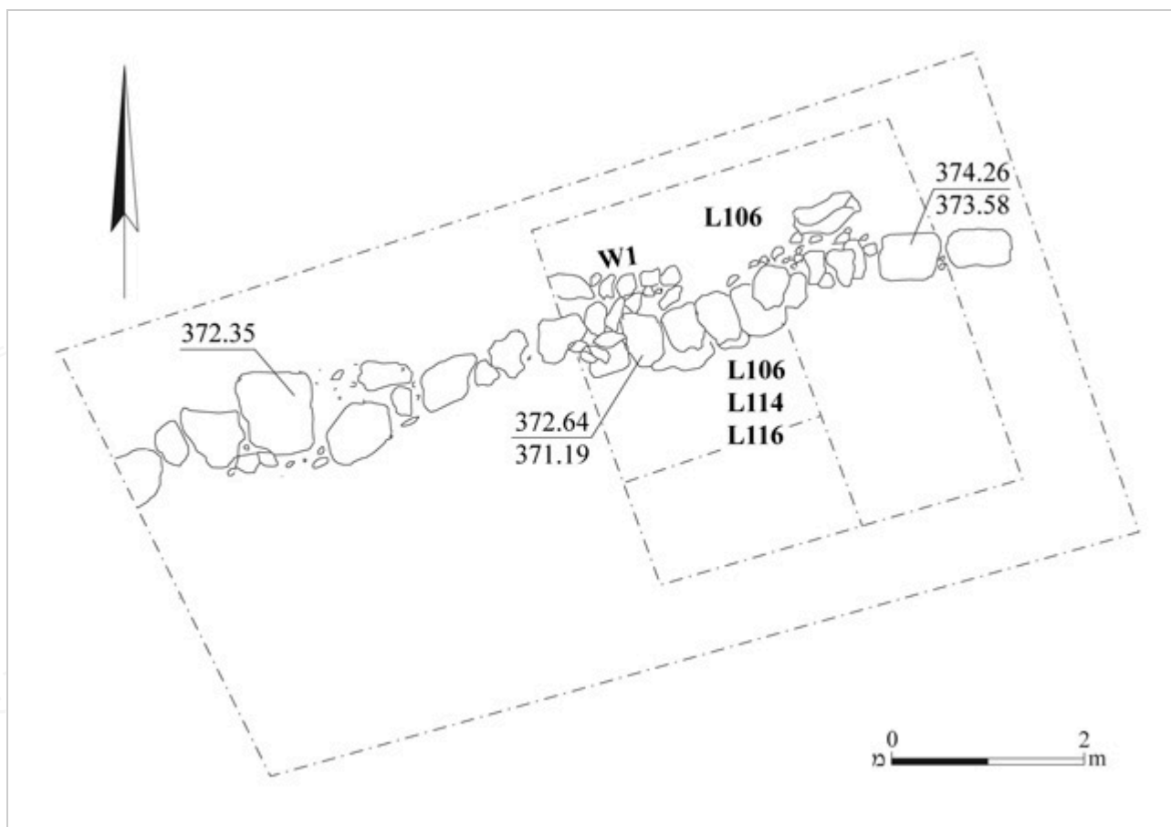
圖 3：F4 農耕圍籬 3 平面圖
