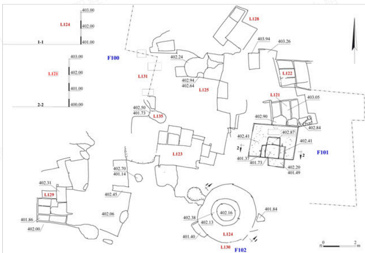
圖 17：B 區，平面圖及剖面
