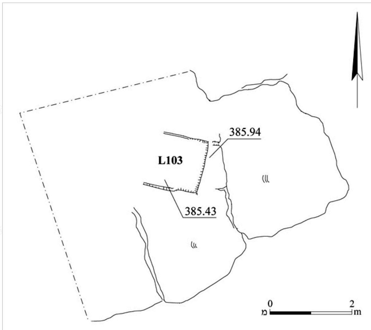
圖 15：F13 採石場，平面圖
