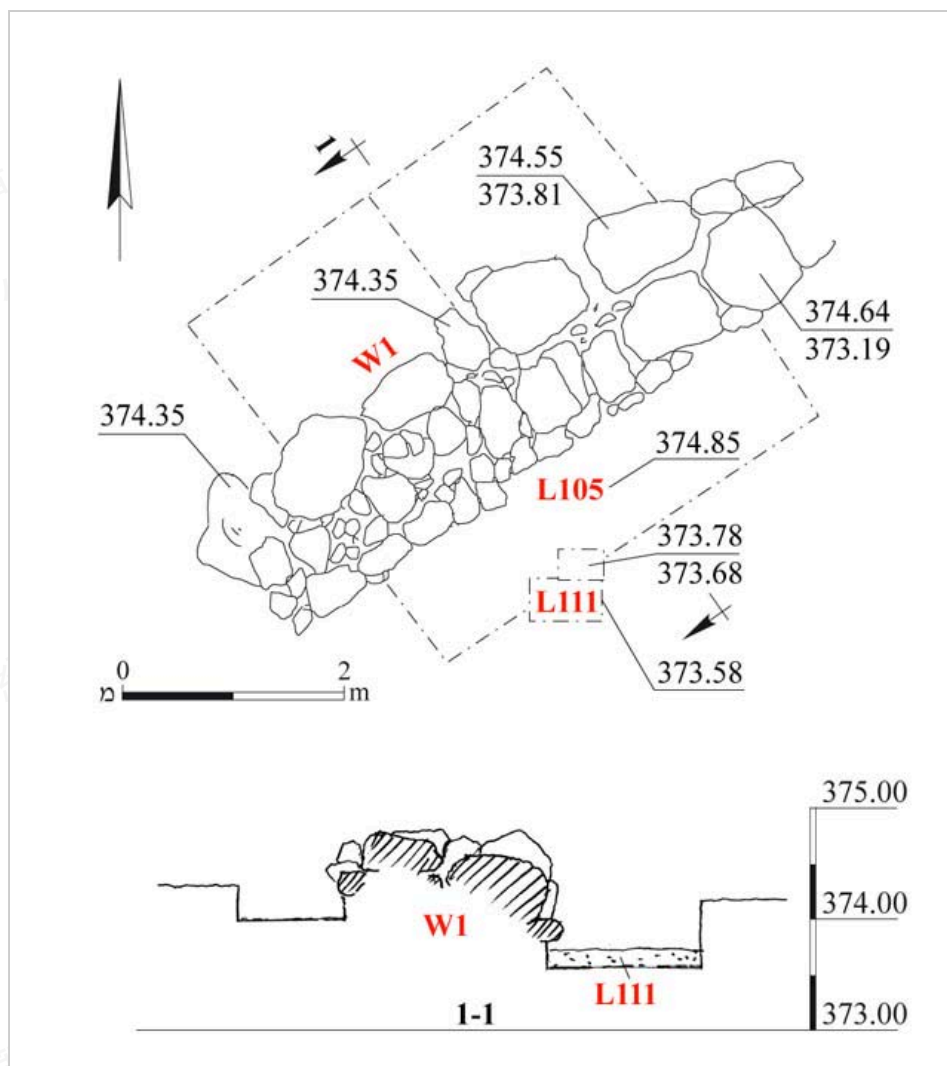
圖 8：F5 牆／水壩，平面圖及剖面
