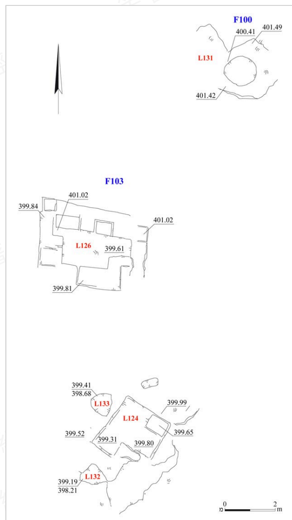
圖 19：F103 平面圖
