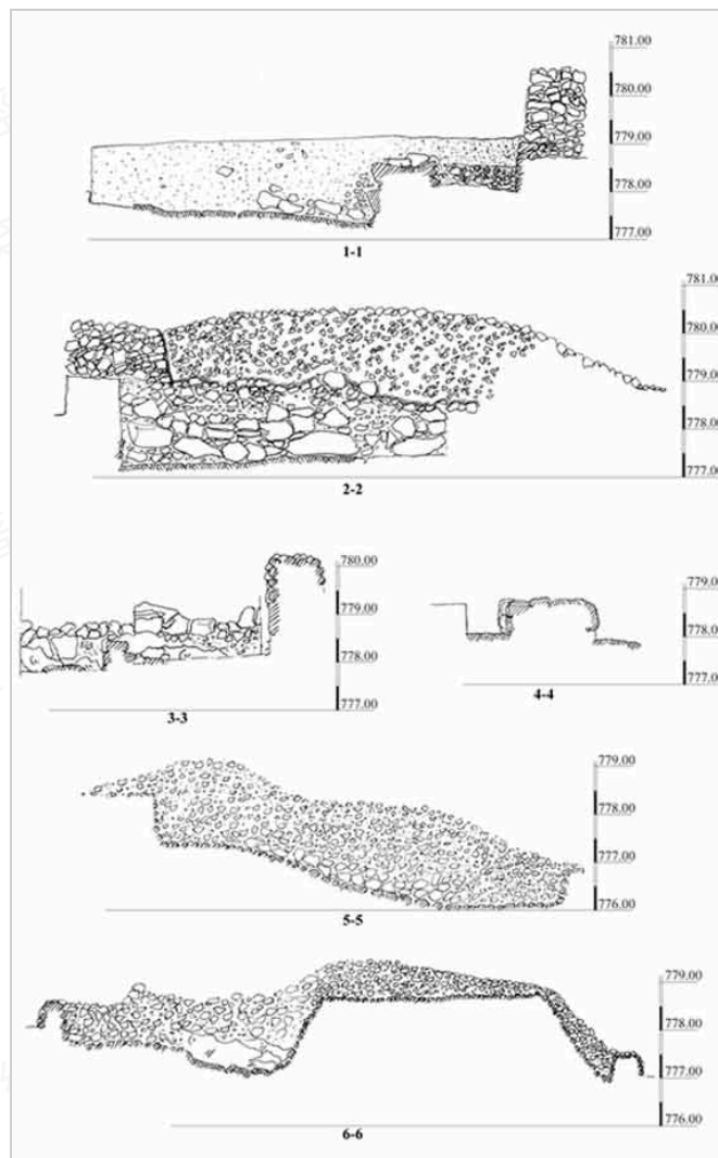
圖 4：剖面圖。
