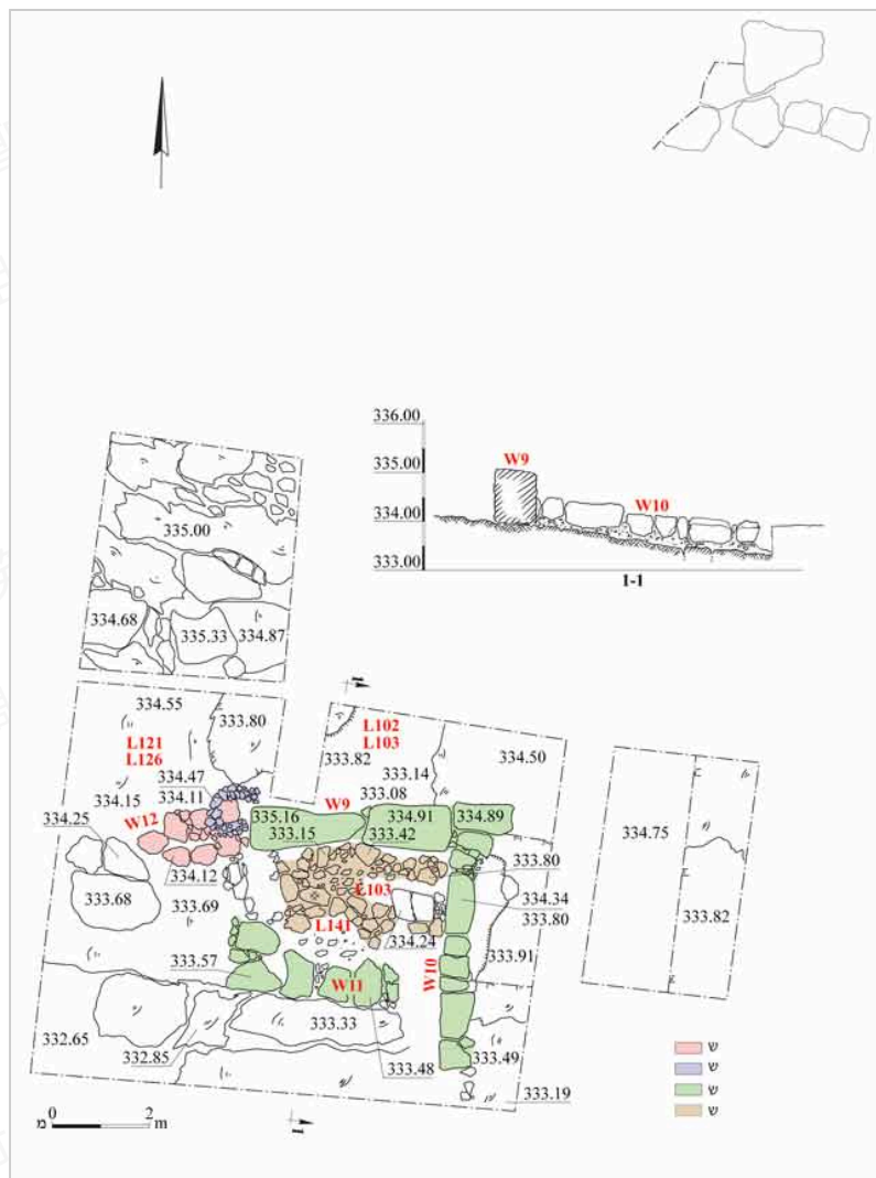
圖 2：平面圖與剖面圖。
