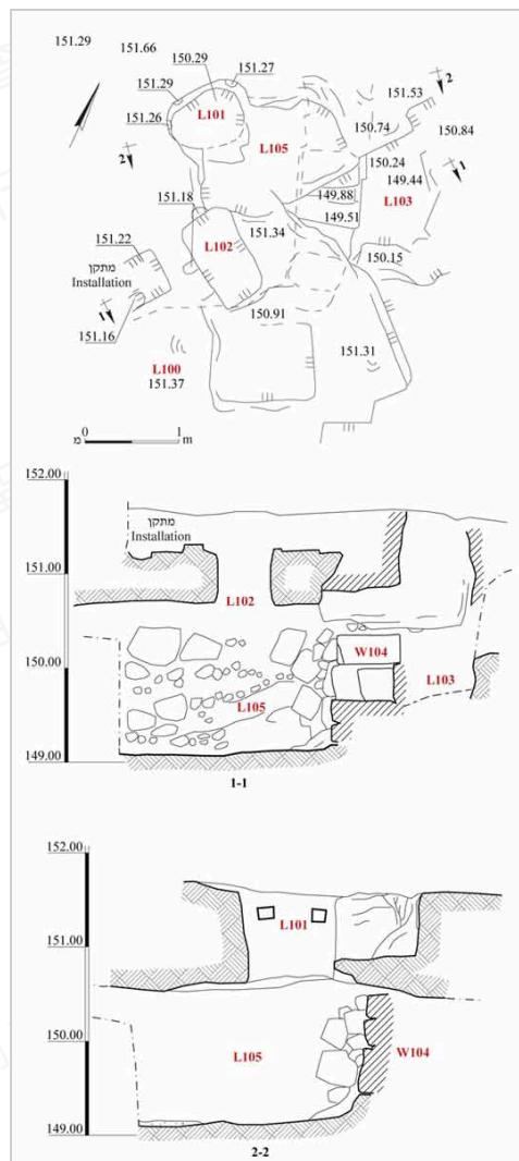
圖 2：平面圖與剖面圖
