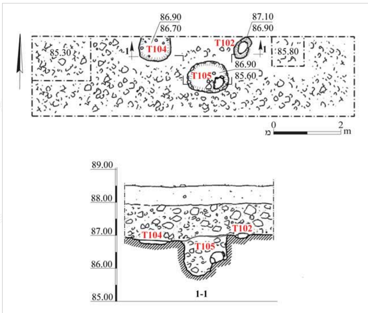
圖 3：平面圖與剖面圖
