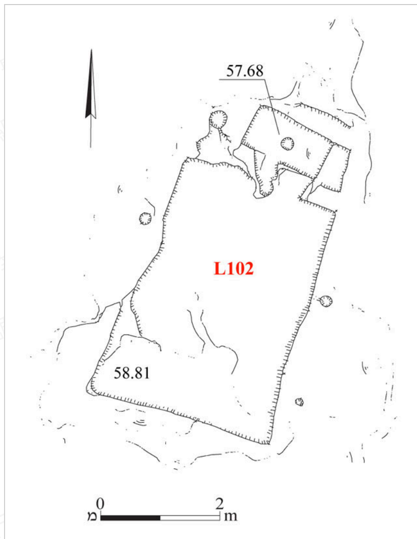
圖 3：榨酒池 102，平面圖。
