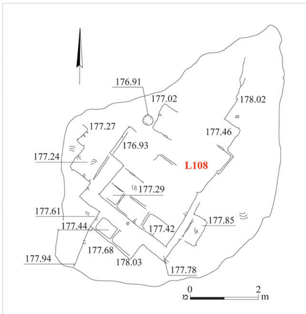
圖 14：採石場 108 平面圖。
