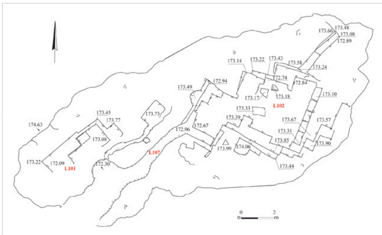
圖 3：採石場 101、102 平面圖。
