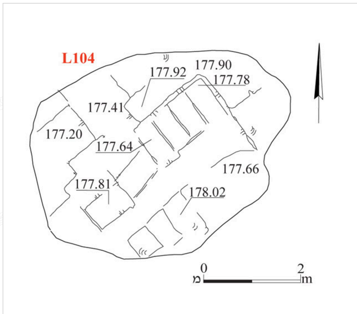
圖 9：採石場 104 平面圖。
