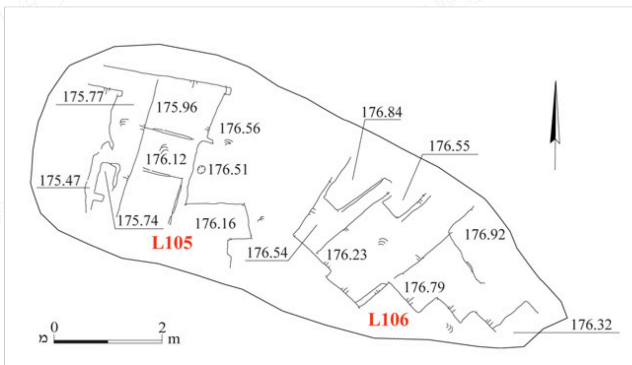
圖 11：採石場 L105、L106 平面圖。
