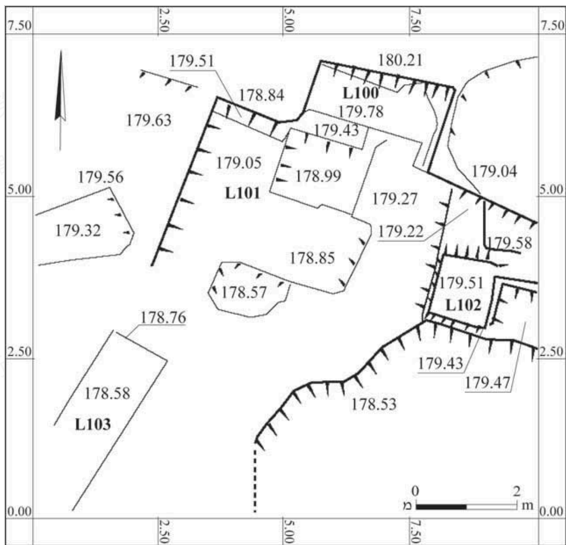
圖 2：採石場，平面圖。
